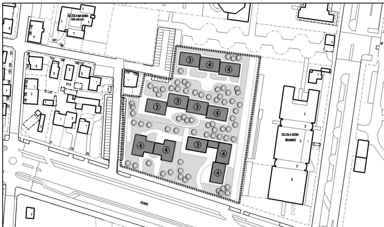
Indicazioni di progetto, planimetria
